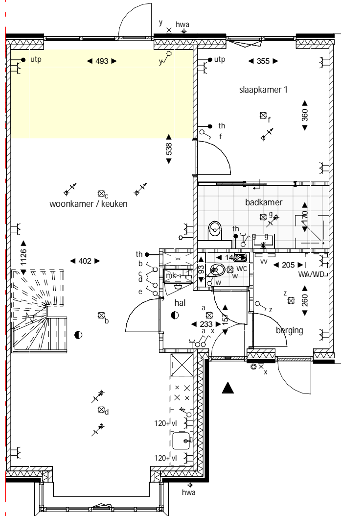
BEGANE GROND - OPTIE: UITBOUW 2,4M
