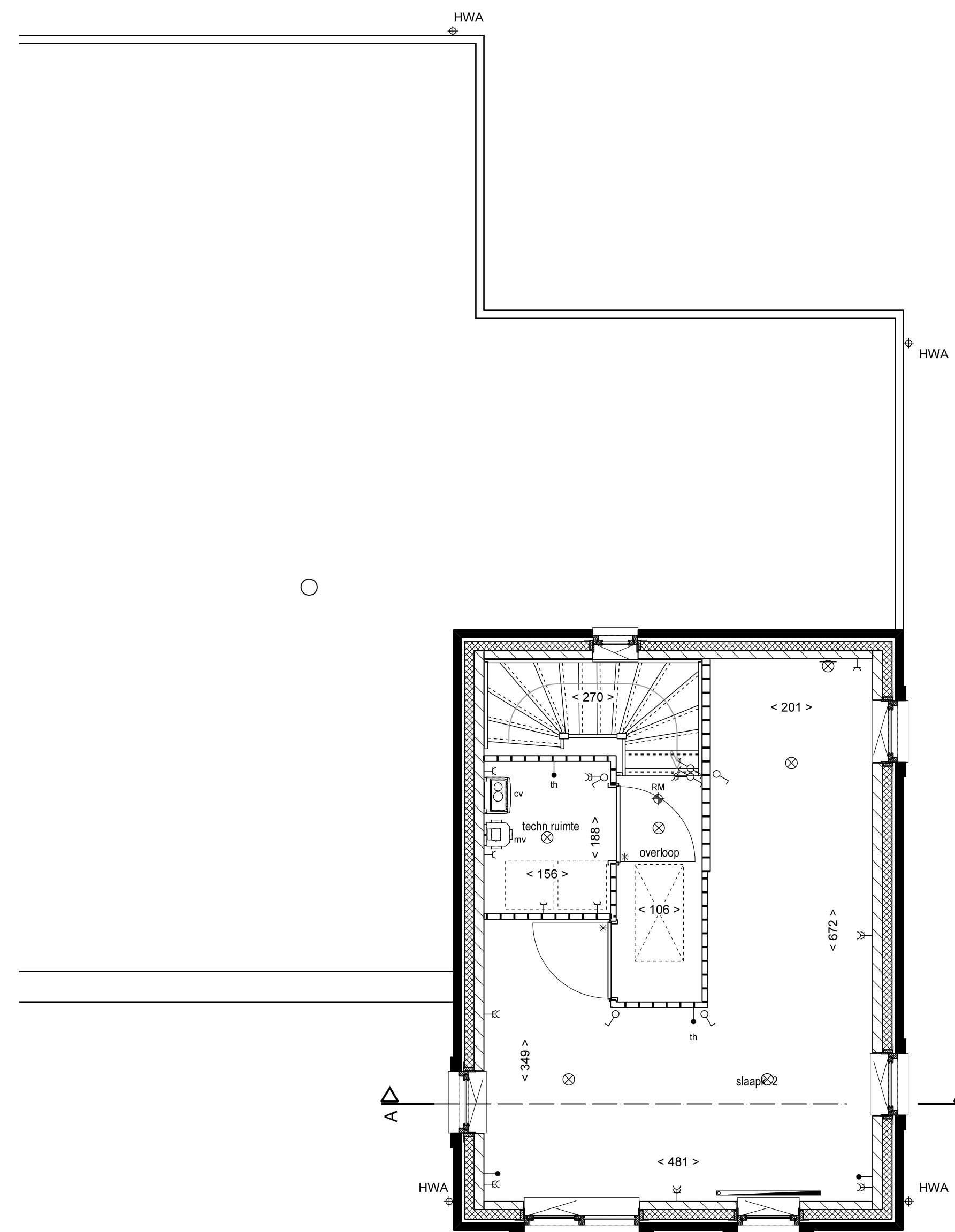
1e VERDIEPING TYPE L1
