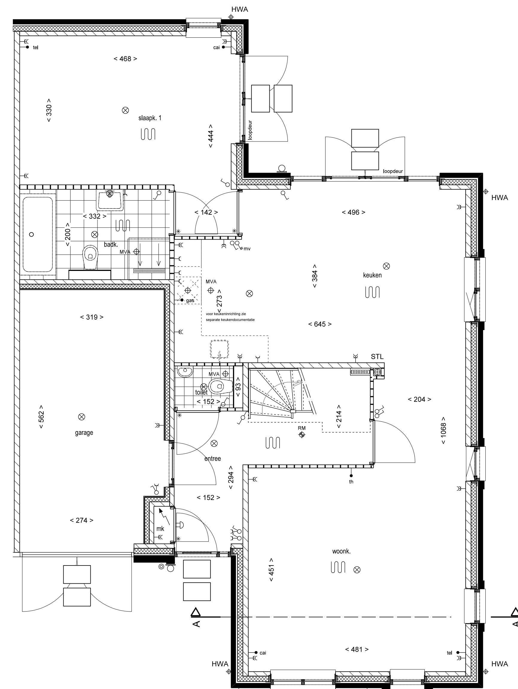
BEGANE GROND TYPE L1
