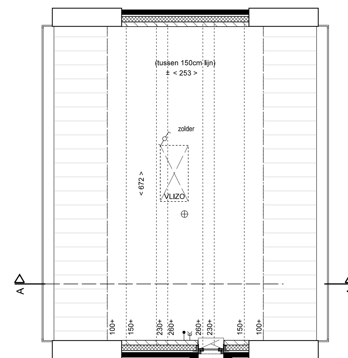
2e VERDIEPING TYPE L1
