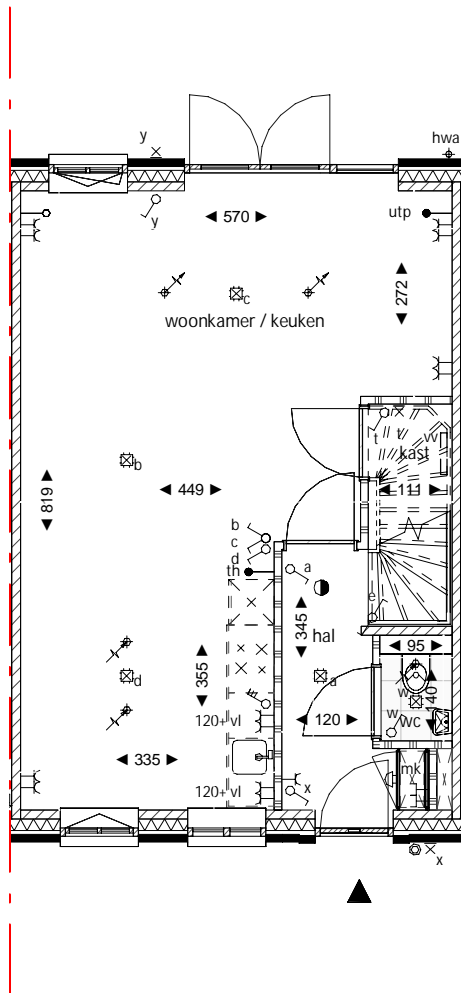
BEGANE GROND - OPTIE: DUBBELE DEUR
