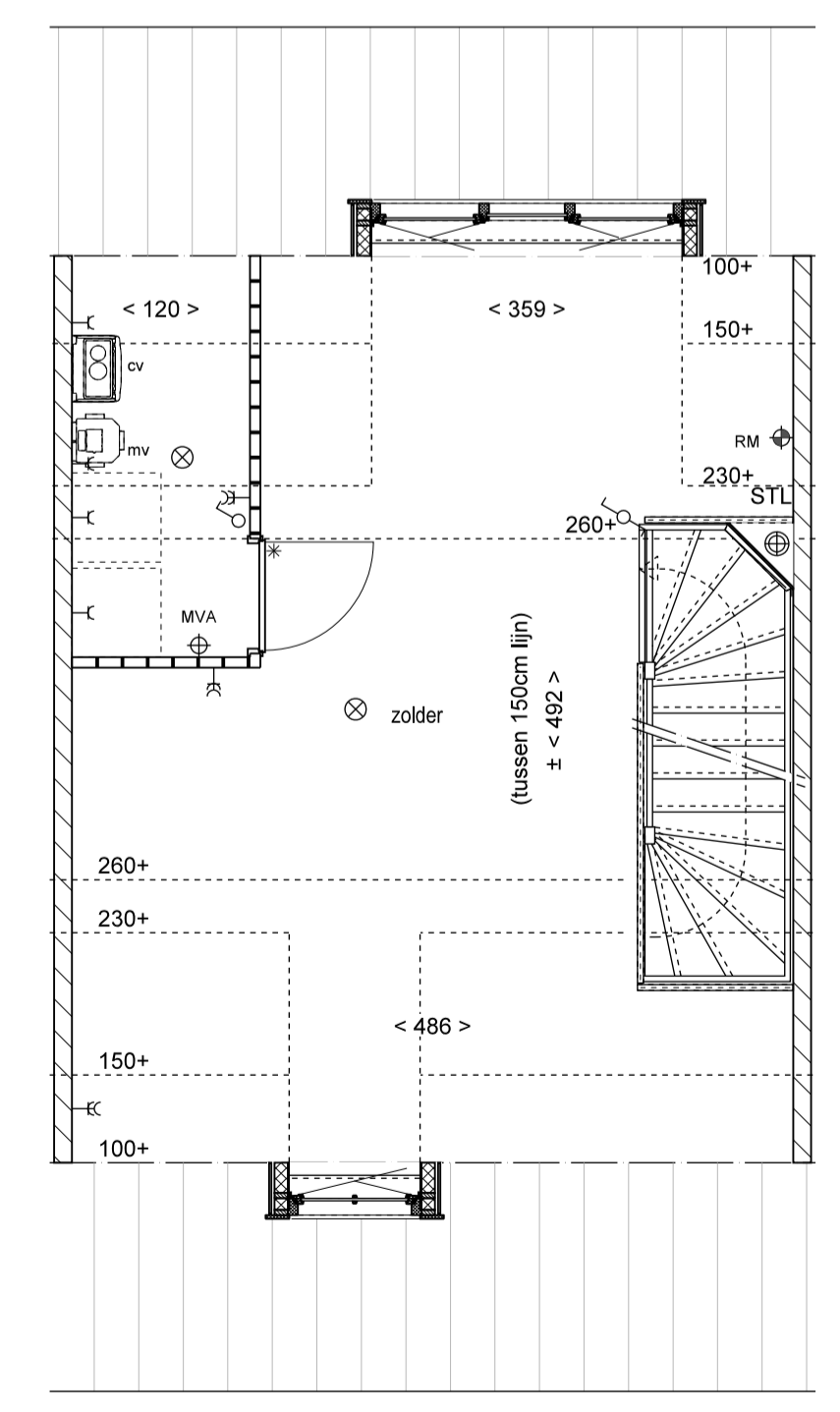
2e VERDIEPING OPTIE: DAKKAPEL VOORGEVEL KLEIN DAKKAPEL ACHTERGEVEL GROOT
