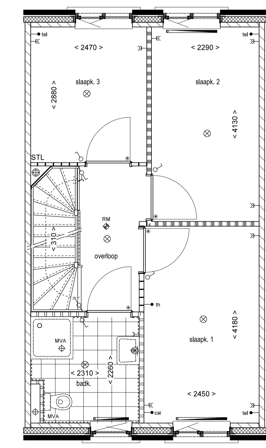
1e VERDIEPING OPTIE: INDELING BADKAMER VOORZIJDE
